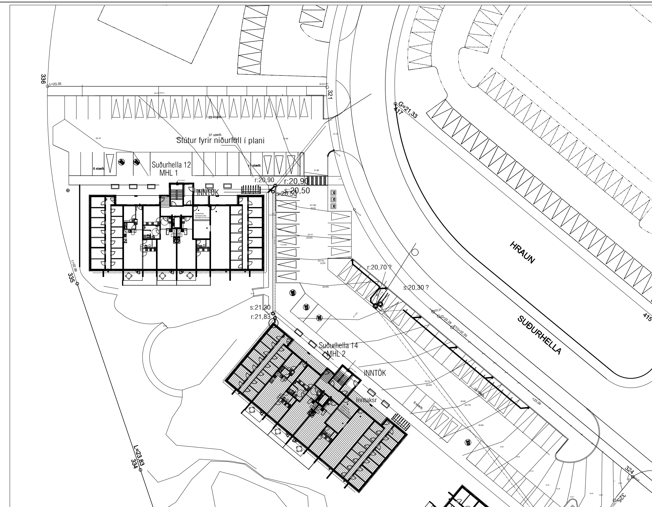
AFSTÖÐUMYND, MKV 1:500
